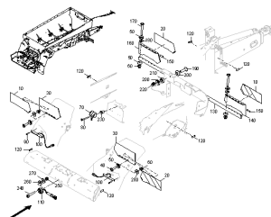
ETB-0000006934, Oświetlenie i oznakowanie
