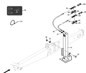
ETB-0000006944, Noga podporowa hydrauliczna
