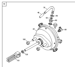
ETB-0000009610, Cylindry membranowe
