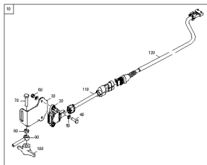
ETB-0000013490, Wspornik czujnika szybkości odchylenia
