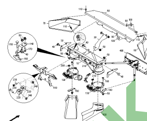
ETB-0000006812, System rozlewania Vario (1)
