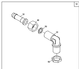
ETB-0000009609, Łącznik kolankowy M22 S13
