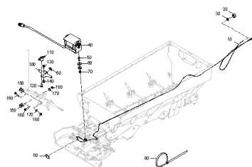
ETB-0000006954, Zestaw mocowania kamery cofania
