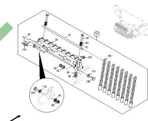
ETB-0000006902, Grabie łańcuchowe
