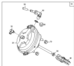
ETB-0000009469, Cylindry membranowe
