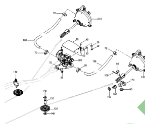
ETB-0000009823, Pneumatyczny układ hamulcowy Typ 36 (2-CZĘŚCI) BKR (2)
