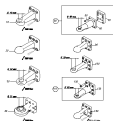
ETB-0000006770, Ucho do ciągnięcia
