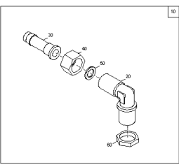
ETB-0000009609, Łącznik kolankowy M22 S13
