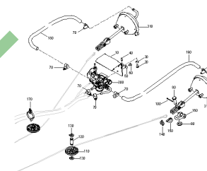
ETB-0000009810, Pneumatyczny układ hamulcowy Typ 30 (2-CZ. BKR) (2)
