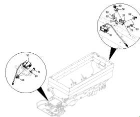
ETB-0000009162, Zestaw kamer
