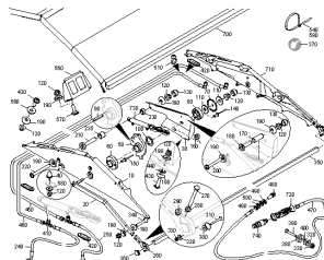
ETB-0000009113, Plandeka hydrauliczna (1)
