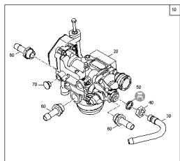
ETB-0000009468, BKR 2-stopniowy
