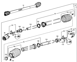
ETB-0000009541, Wałek przegubowo-teleskopowy EJ673
