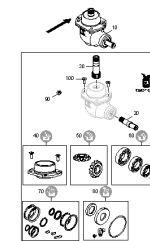
ETB-0000011531, Zewnętrzna mechaniczna skrzynia biegów
