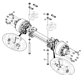
ETB-0000006801, Oś: Sztywno hamowana
