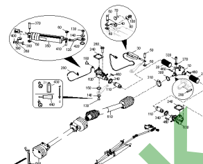
ETB-0000006967, Napęd Tronic z Auto-TS RE. i Flowcontrol
