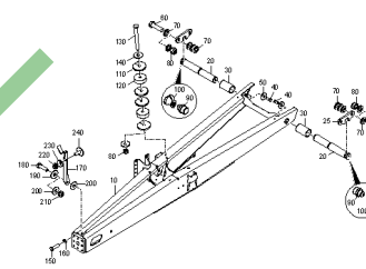
ETB-0000010257, Zaczep dolny 4 t
