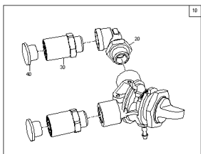
ETB-0000009464, Zawór 3/2-drogowy
