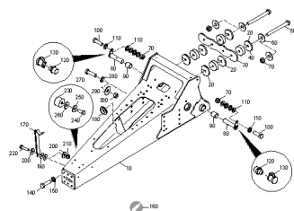
ETB-0000009148, Zaczep dolny Special
