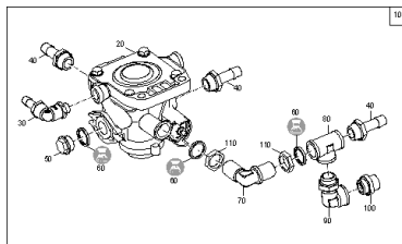
ETB-0000009465, Zawór hamulcowy przyczepy
