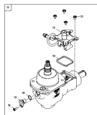
ETB-0000012092, Skrzynia biegów: mechaniczna, kontrola
