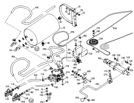
ETB-0000009822, Pneumatyczny układ hamulcowy Typ 36 (2-CZĘŚCI) BKR (1)
