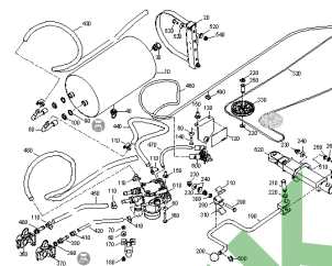
ETB-0000009809, Pneumatyczny układ hamulcowy Typ 30 (2-CZ. BKR) (1)
