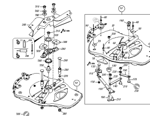
ETB-0000007730, Płyta główna po lewej stronie z ClickTS
