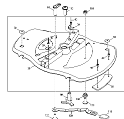
ETB-0000007475, Płyta główna Click-TS
