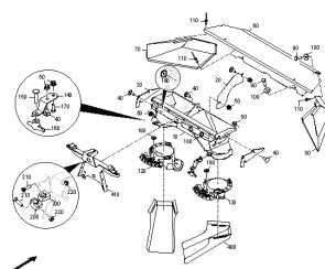
ETB-0000006811, Mechanika rozsiewu
