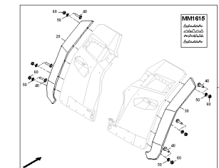
ETB-0000013481, Zestaw montażowy poszerzenia błotnika
