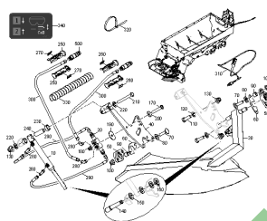
ETB-0000006861, Urządzenie do rozsiewania wapna na granicy
