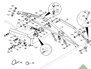
ETB-0000009118, Plandeka hydrauliczna (2)
