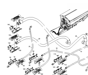
ETB-0000010798, Węże hydrauliczne US / CA
