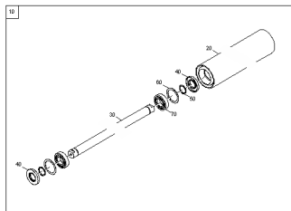
ETB-0000011083, Bęben odchylający
