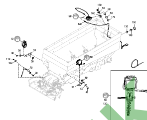
ETB-0000006936, Oświetlenie robocze
