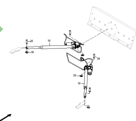
ETB-0000006813, Rozsiewacz vario(2)
