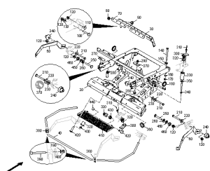
ETB-0000006776, Belki rozrzutnika
