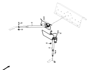
ETB-0000006813, Rozsiewacz vario(2)
