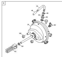
ETB-0000009610, Cylindry membranowe
