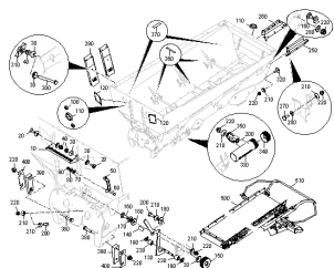
ETB-0000006758, Podstawowa rama/skrzynia maszyny
