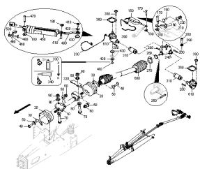
ETB-0000006966, Napęd Tronic z Auto-TS RE.
