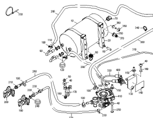
ETB-0000009412, Pneumatyczny układ hamulcowy typu 36
