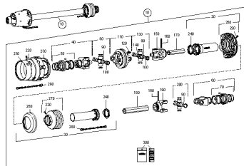
ETB-0000006985, Wałek przegubowo-teleskopowy EJ679 - 1360 mm 1 3/8 cala, 8x32x38, z widelcem Russia
