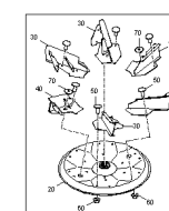
ETB-0000006813, Rozsiewacz vario(2)
