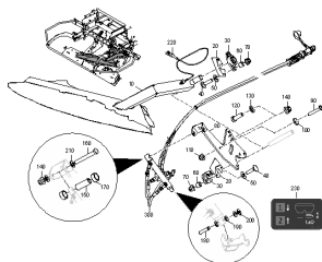
ETB-0000006859, Urządzenie do rozrzucania granic
