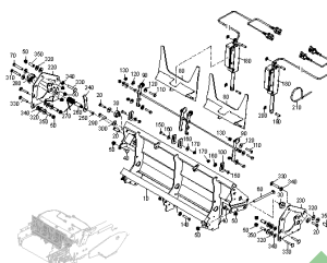
ETB-0000006898, Jednostka z podwójnym suwakiem
