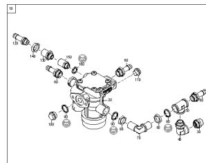
ETB-0000011806, Ciagniony zawór hamulcowy
