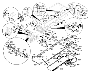
ETB-0000009521, Maszyna podstawowa ZG-TX Special
