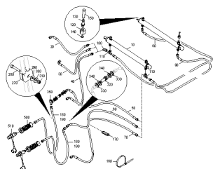
ETB-0000006833, Plandeka uchylna hydrauliczna
